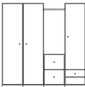
W 190.4 cm H 186.4/70.4 cm Plinth 7 cm
